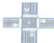
非机动车禁驶区标线
