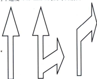
行车速度在60-80 km/h时的导向箭头 及行车速度 \geq 100 km/h时的导向箭头
