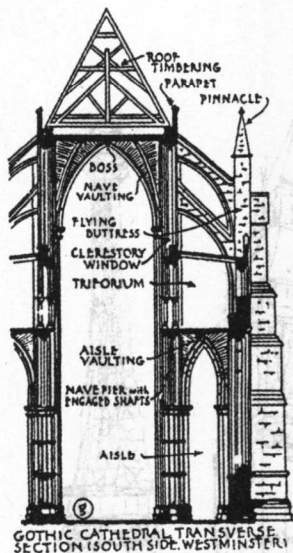
英格兰威斯特敏斯特修道院横断面显示尖券拱上的三角形木屋架。
