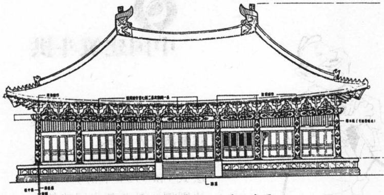
宋“营造法式”立面设计示意图
