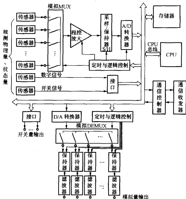
图 1-1 微型计算机系统框图
