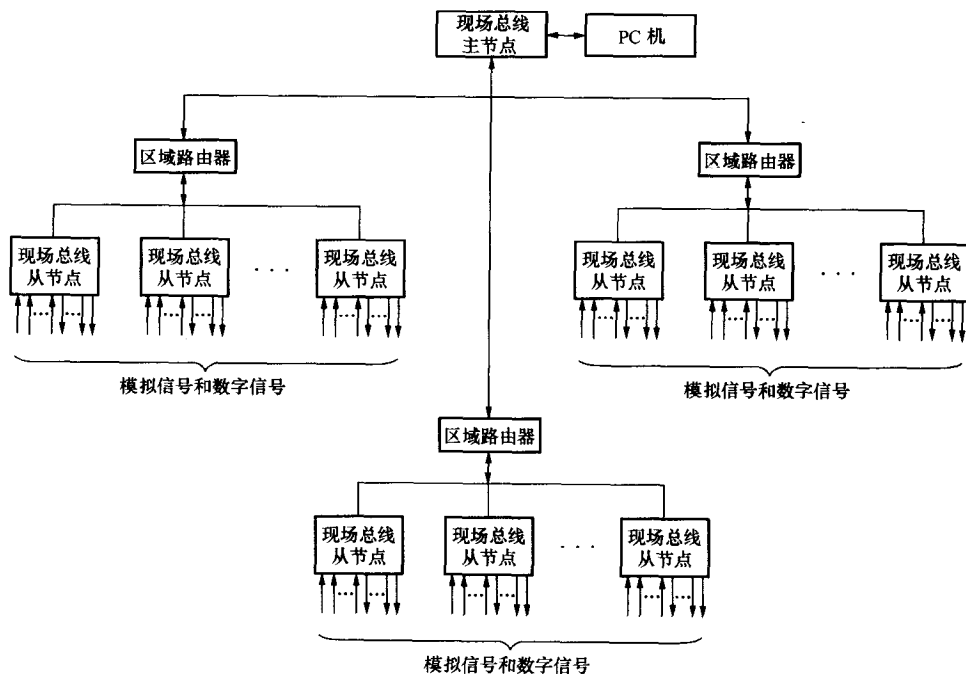
图 1-5 现场总线系统结构框图
