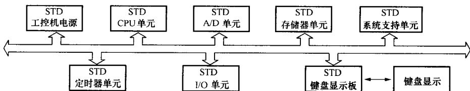
图 1-3 STD 总线工业控制机结构示意图
