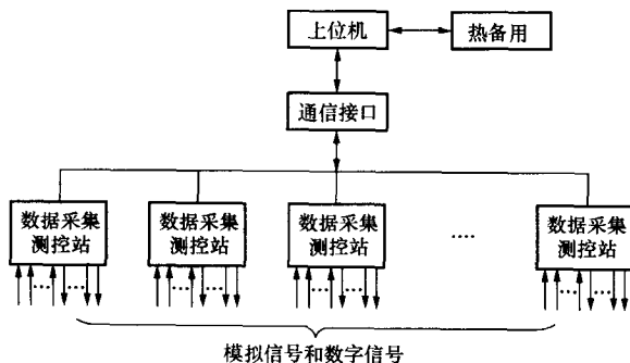
图 1-4 集散系统结构框图
