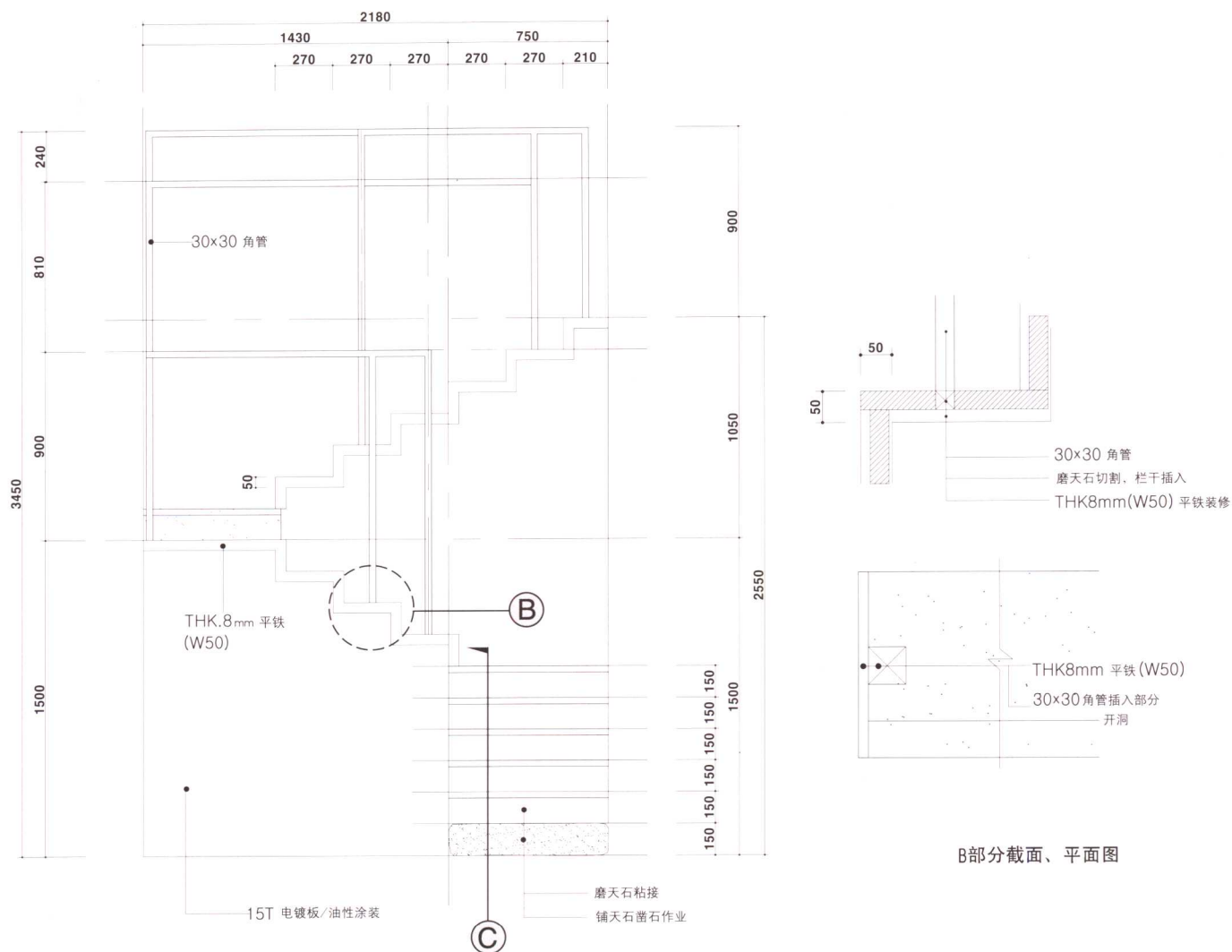
阶梯立面详细图
