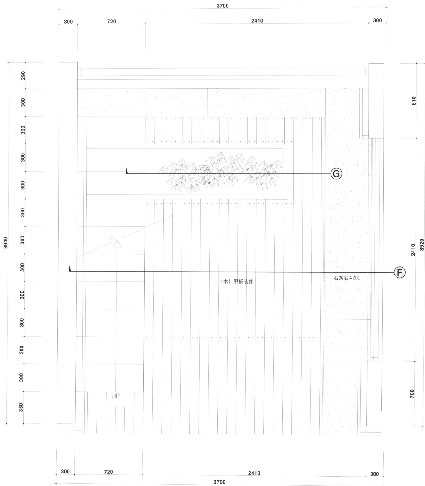
4层中庭平面图
