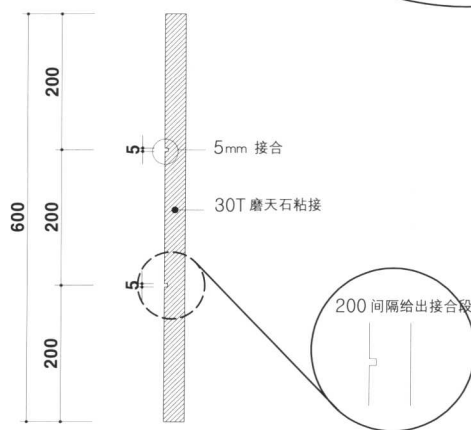
磨天石施工
