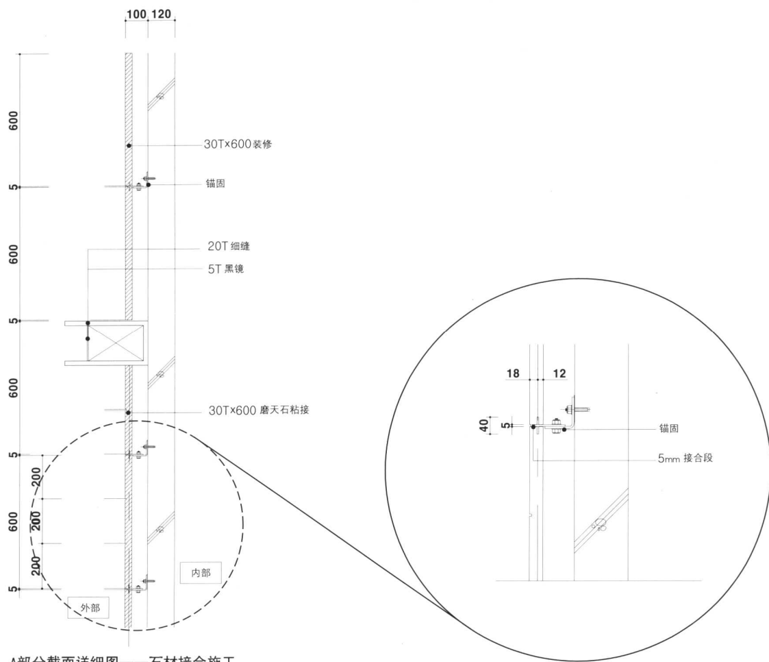
A部分截面详细图——石材接合施工
