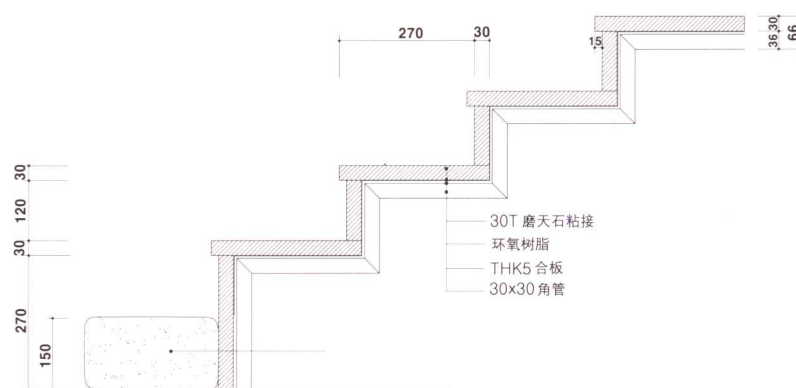
C部分截面图
