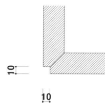
外角部分施工
