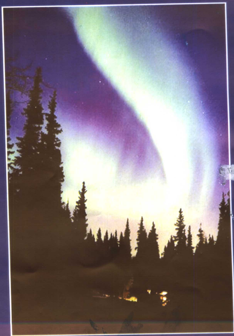
形状怪异的极光
