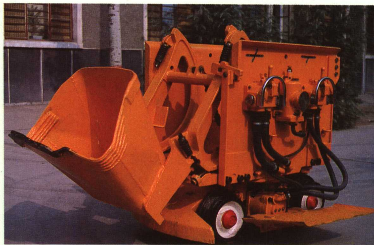
装岩机
