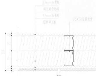
大法庭大样 7
