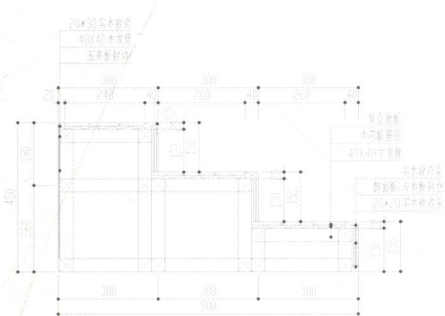
大法庭大样 1
