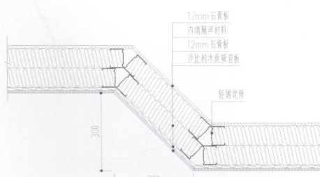
大法庭大样 5
