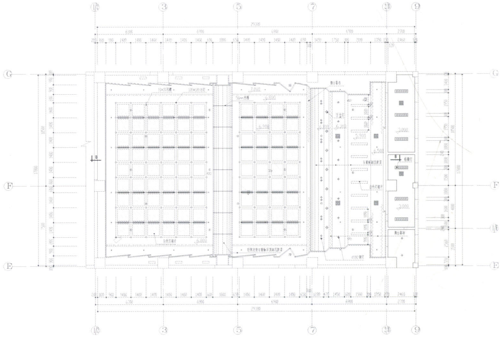
大法庭天花图
