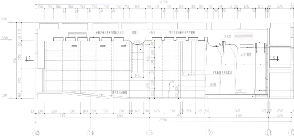
大法庭A立面图
