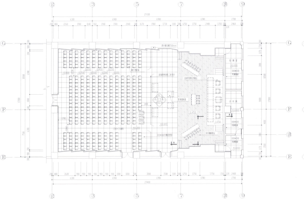
大法庭平面图
