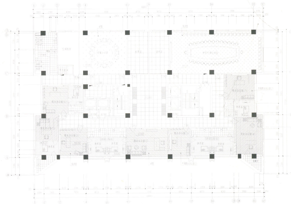
10层平面图
