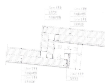
大法庭大样 4
