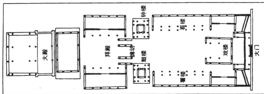
山西会馆总平面图
