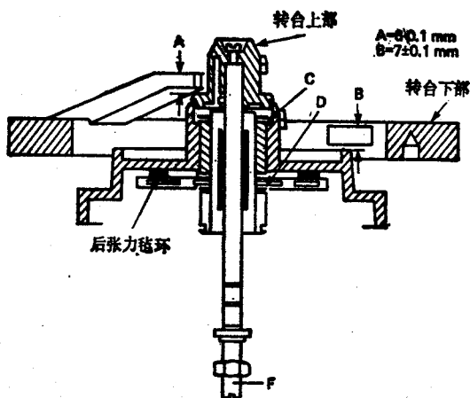
图 1·3 带盘载体装置
