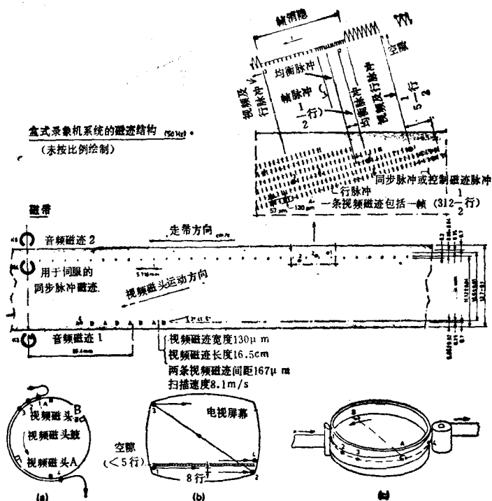
图 1-4 N1500 机器的记录磁迹
