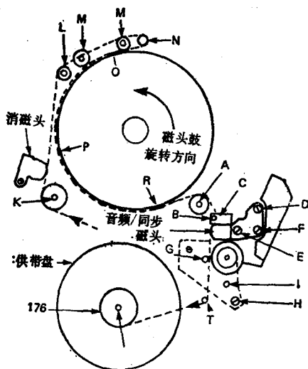
图 1·1 飞利浦N1500的带路
