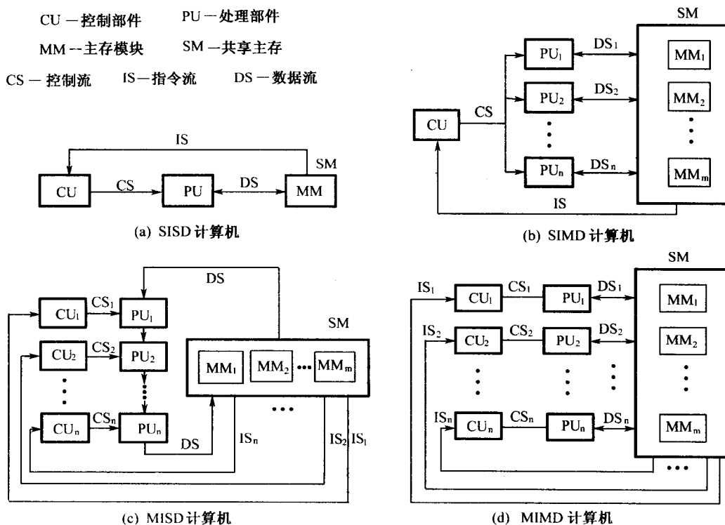
图 1.2 Flynn 分类法的 4 类机器结构
