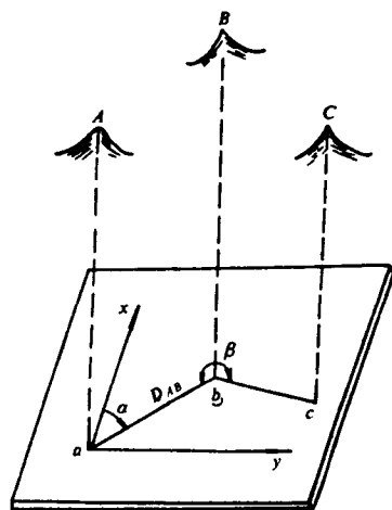
图 1-5 地面点的相对位置
