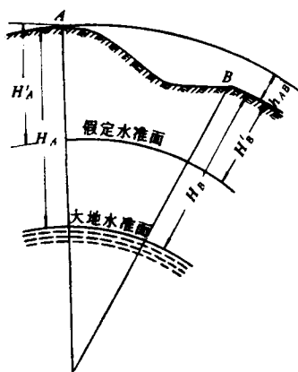
图 1-4 绝对高程与相对高程
