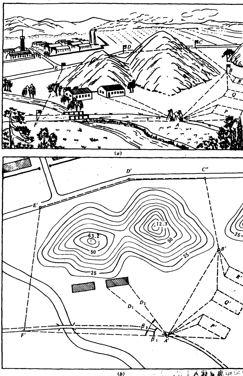
图 1-7 测图原则示意图
