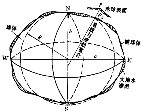
图 1-1 大地水准面与椭球体
