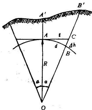
图 1-6 用水平面代替水准面
