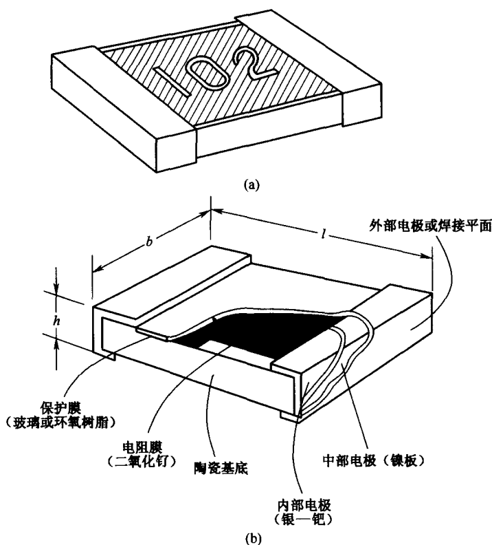
图 1-1 矩形片状电阻的外形
