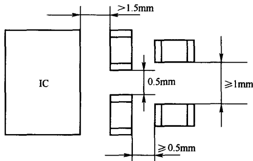
图 1-4 片状电阻的间距要求
