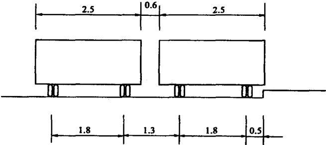
图 1-1-2 车辆荷载横向布置 (图中尺寸单位为 m)
