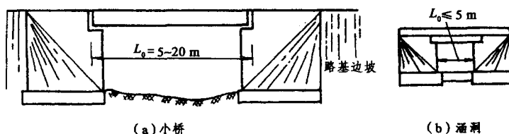
图 1-1-5 桥涵
