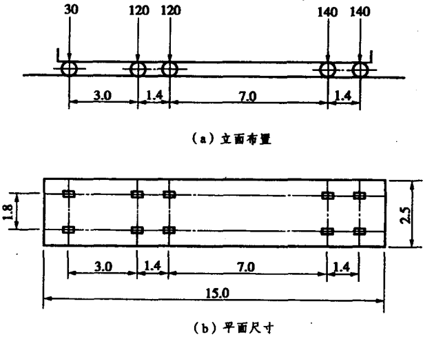
图 1-1-1 车辆荷载的立面、平面尺寸 (图中尺寸单位为 m，荷载单位为 kN)
