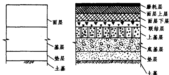
图 1-1-4 路面
