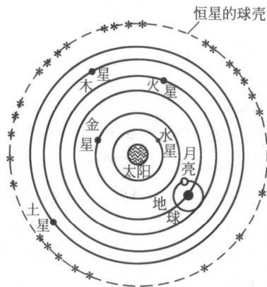
图 1-2 哥白尼关于宇宙格局的日心理论图
