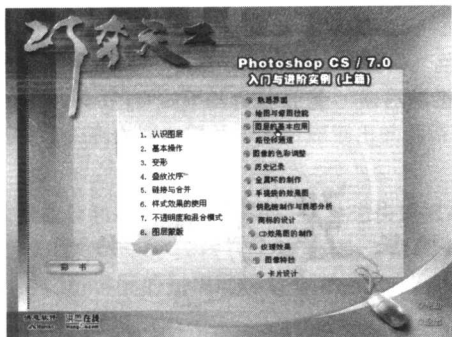
图 1 程序主界面
