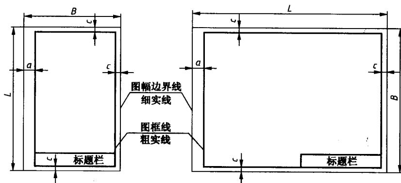
图 1-9 留有装订边的图纸格式
