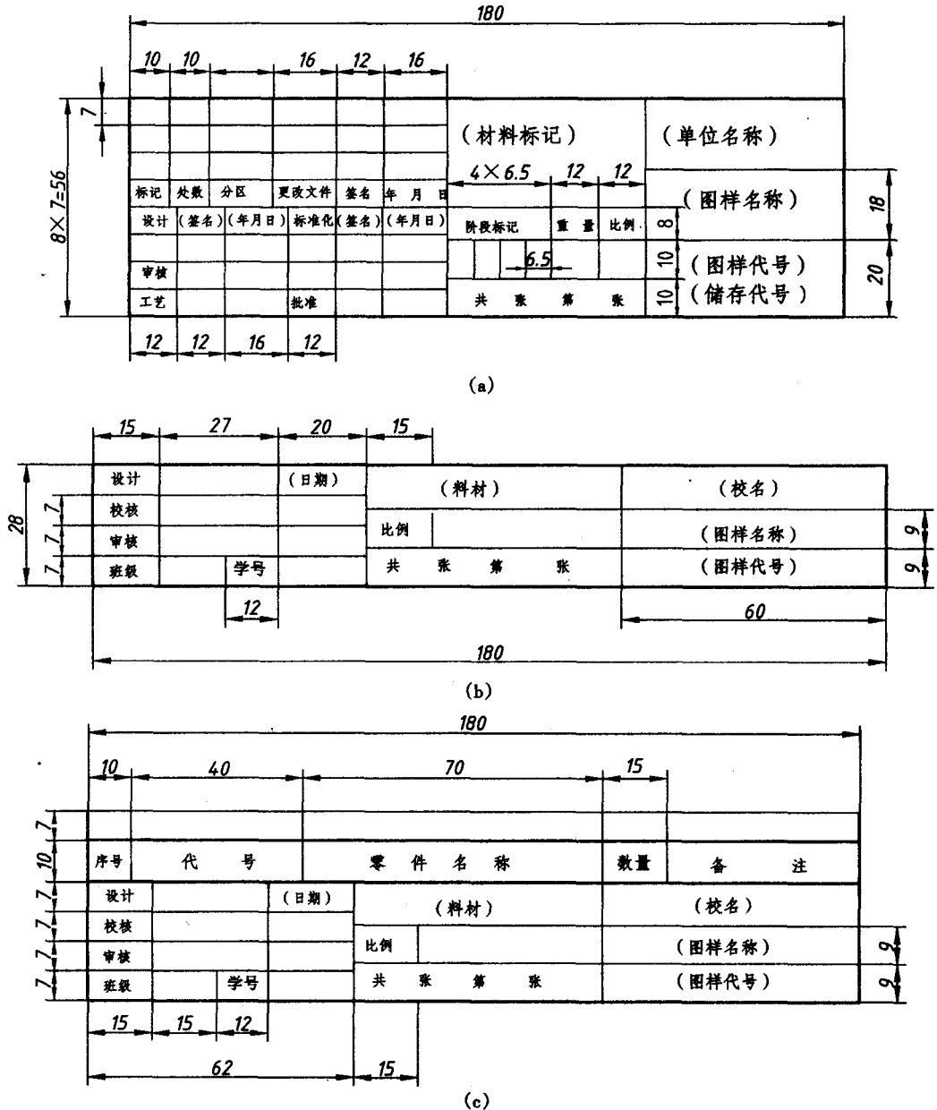
图 1-11 标题栏的格式
