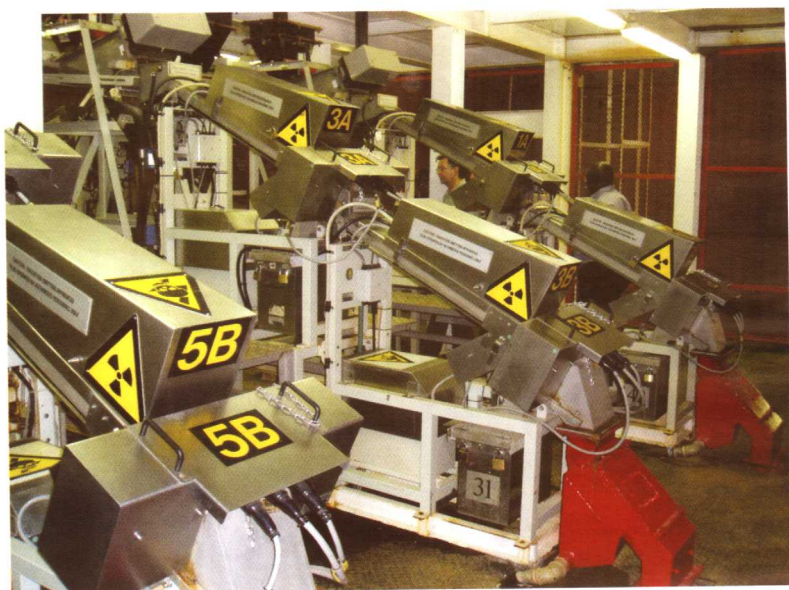
图5-3 X射线选矿(梁伟章摄影)
