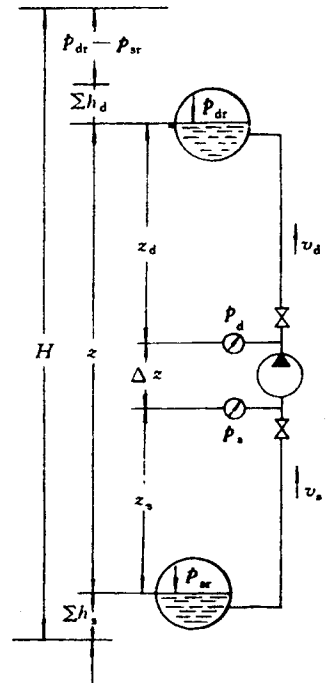
图 0-1 泵装置简图
