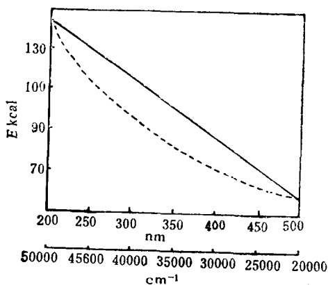
图 1.2 能量和波数及波长的关系 ——能量和波数; ——能量和波长。
