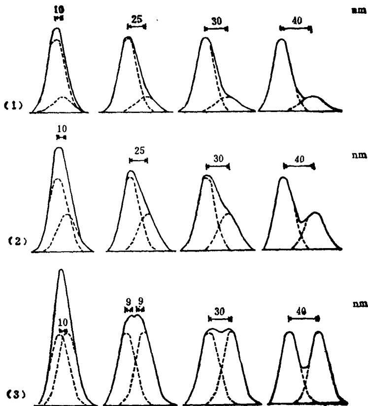
图 1.6 重叠的吸收带
