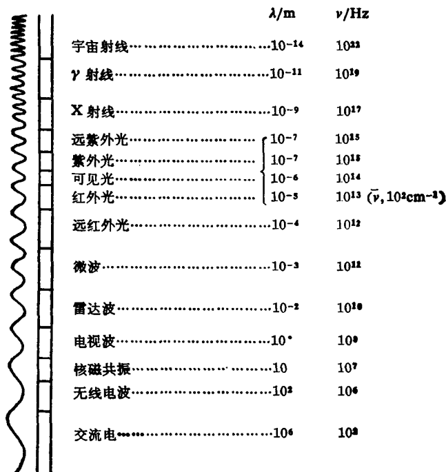
图 1.1 电磁波谱示意图
