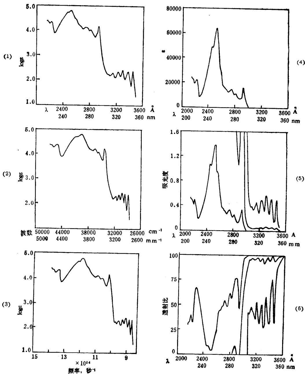
图 1.5 萘的紫外吸收光谱(不同表示方法)
