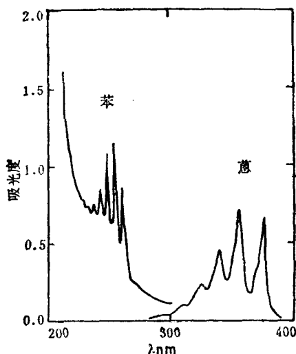
图 1.3(a) 苯和葱的 {}^1L_b 带(溶剂 环己烷)
