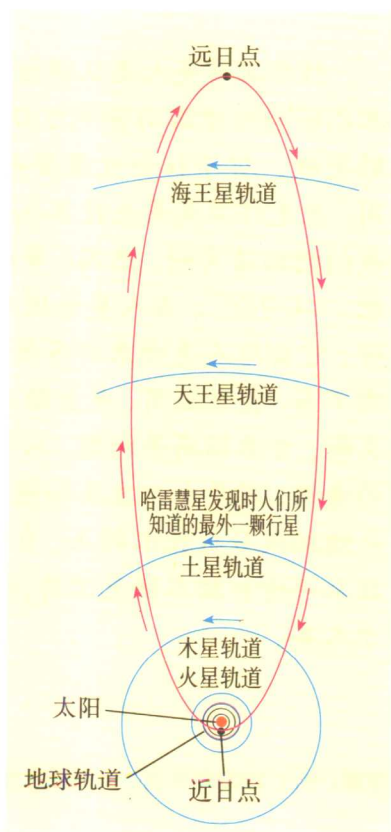
图0-13 甲 哈雷彗星和它的公转轨道。公元前613~1910年，中国有它31次回归的记录。1705年，英国天文学家哈雷根据牛顿的万有引力定律正确地预言了它的回归。
