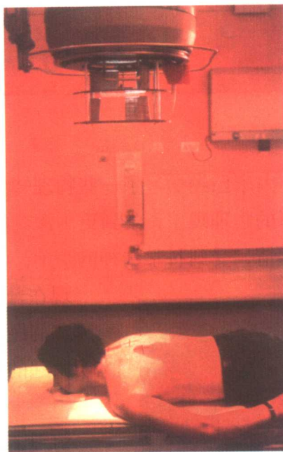
图0-3 患肿瘤的病人在接受放射治疗
