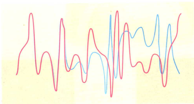
图0-13 丙 单变量数值仿真。洛伦兹 ① 将仅仅相差0.000 1的两个初始条件输入一个数学方程,计算得出的两条曲线不久就分道扬镳,南辕北辙。真是“差之毫厘,谬以千里”。
