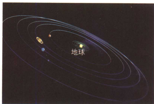
图0-12 乙 16 世纪，人们认 识到地球和几 大行星都在绕 太阳运动。
