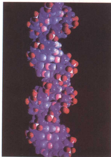
图0-8 脱氧核糖核酸的双螺旋结构模型
