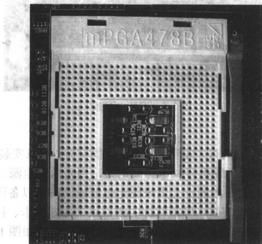
图 1-3 CPU 插座图
