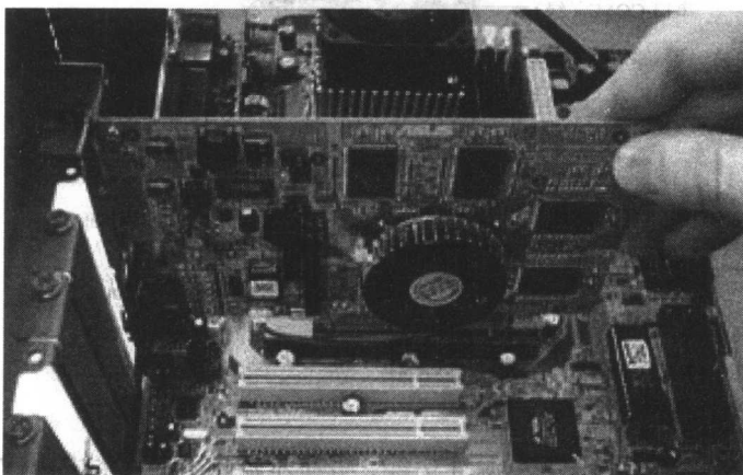
图 1-13 显卡安装
