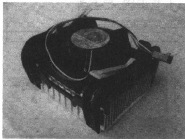
图 1-4 CPU 风扇
