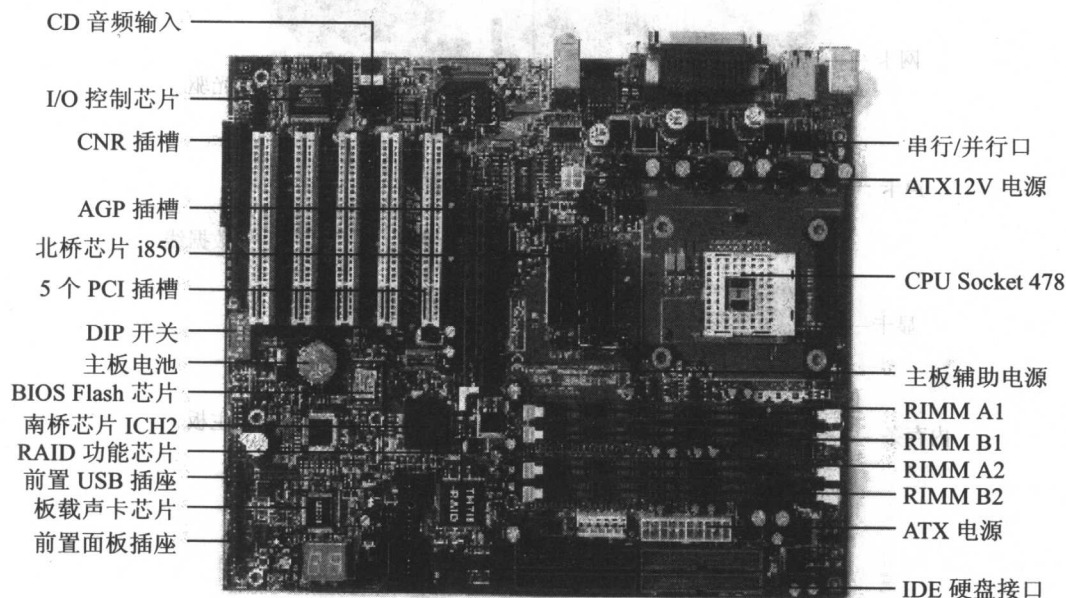
图 1-2 主板结构图
