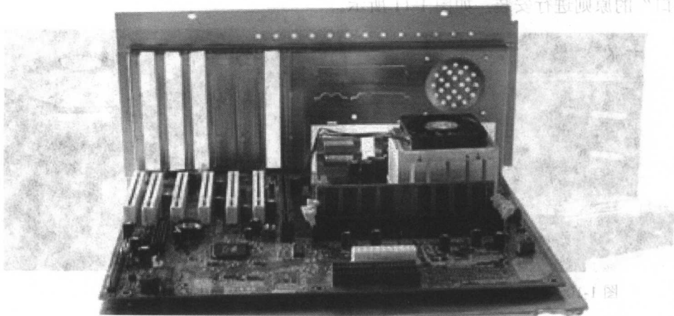
图 1-8 主板安装
