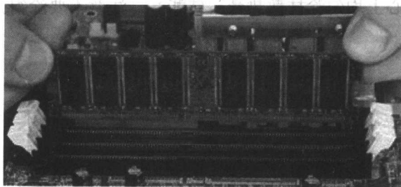
图 1-5 安装内存条
