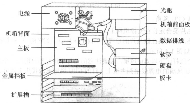
图 1-6 机箱内结构示意图
