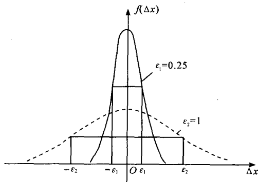
图 1.2 正态分布曲线
