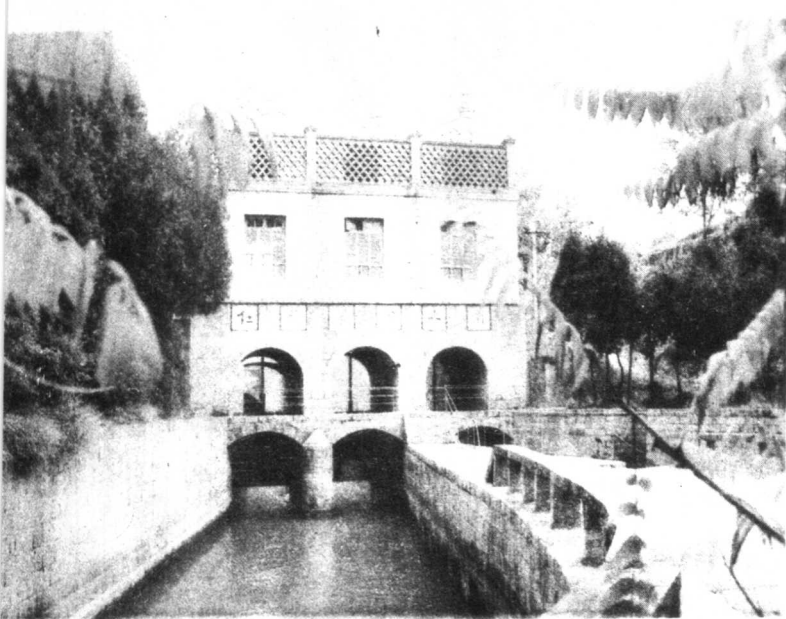
总干渠分水岭分水闸
