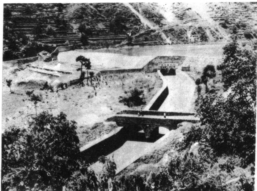
白家庄双拱形空心坝
