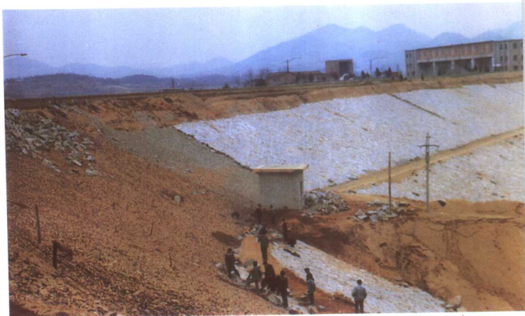
主坝河槽左段 加固施工
