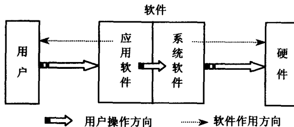
图 1-2 软件的作用
