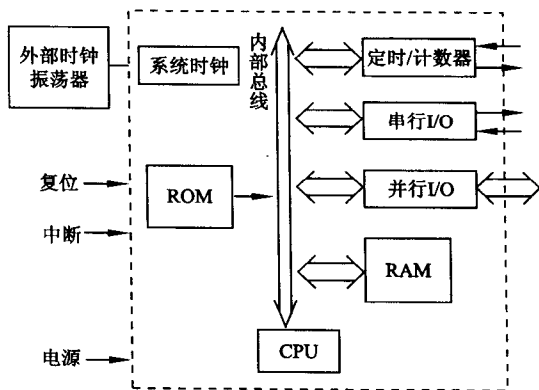
图 1-1 典型单片机的基本构成
