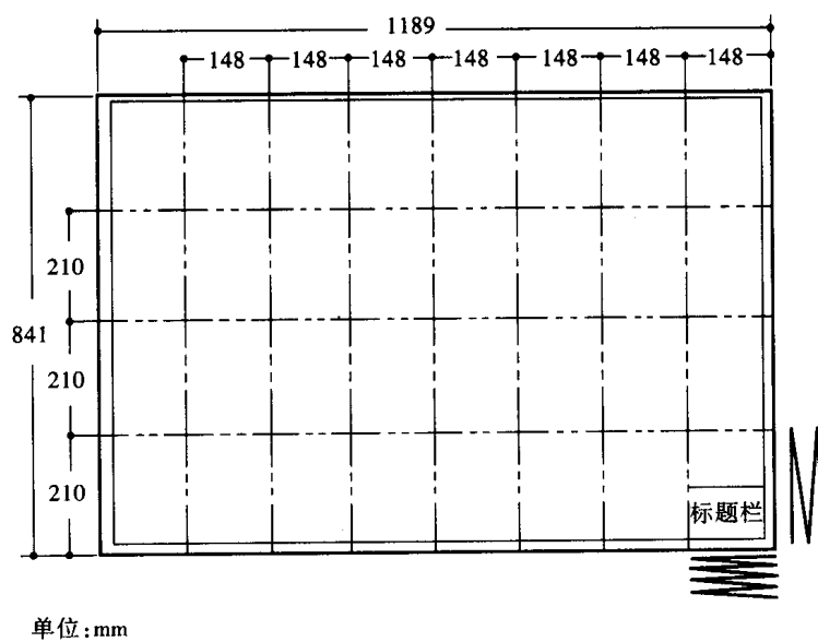
图 1-3 0 号图纸折叠形式
