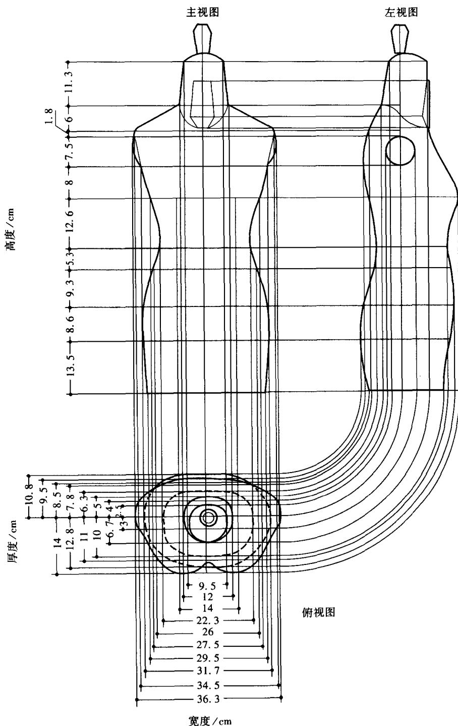
图 1-4 工业用身型模台三视图
