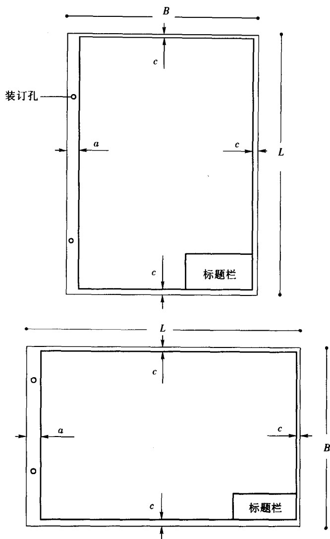
图 1-1 图纸格式
