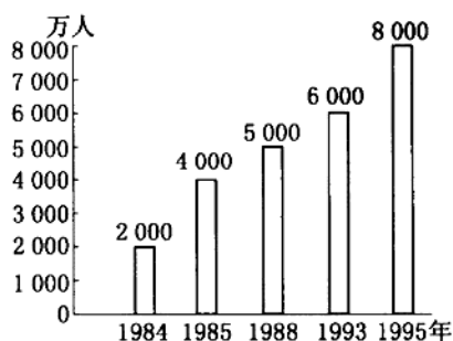
图 14 20 世纪 80 年代中期以后我国人口迁移和流动人口数量变化图
