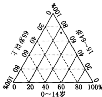
图 13 人口年龄构成的比重图
