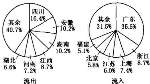
图8 2001年我国跨省流动人口地区构成
