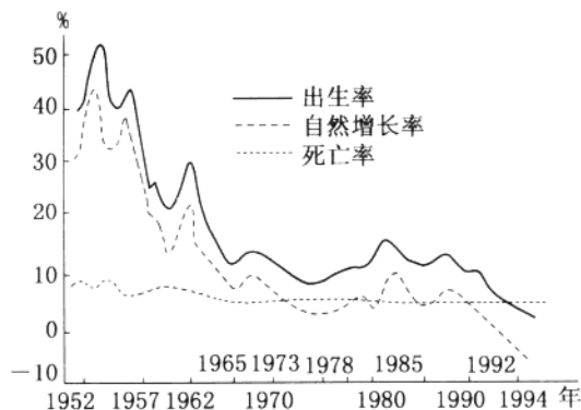
图 16 上海市人口出生率、死亡率和自然增长率图
