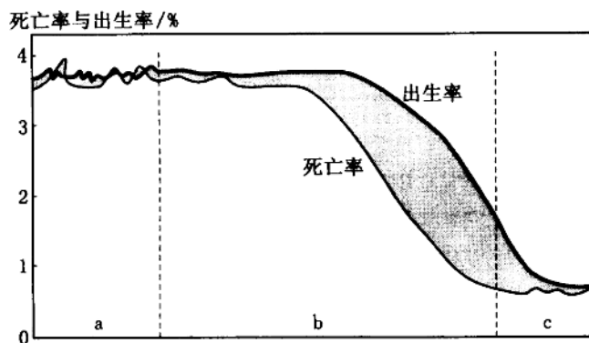
图 5 人口增长模式及其转变示意图
