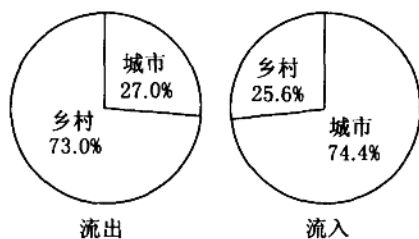
图9 2001年我国流动人口城乡结构
