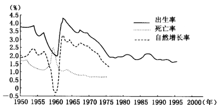
图6 我国人口出生率、死亡率、人口自然增长率的发展变化图
