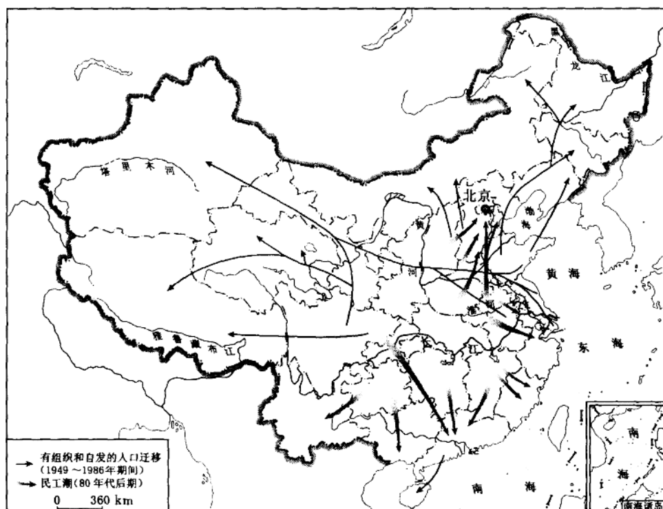
图 12 1949 年以来我国国内人口迁移的主要流向图
