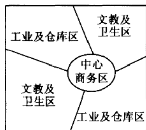
图 19 某城市地域结构模式图
