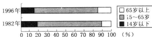
图 17 1982 年与 1996 年上海市年龄构成比较图
