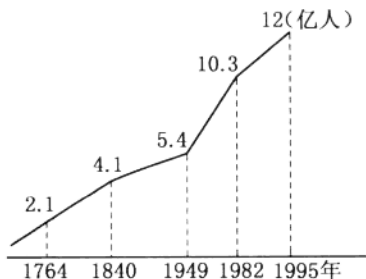
图 18 我国人口增长示意图
