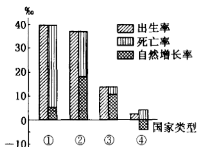
图 2 四种类型国家的人口增长示意图
