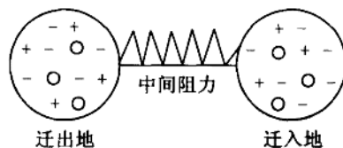
图10 人口迁移的拉力和推力示意图
