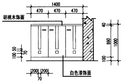
鞋柜立面图
