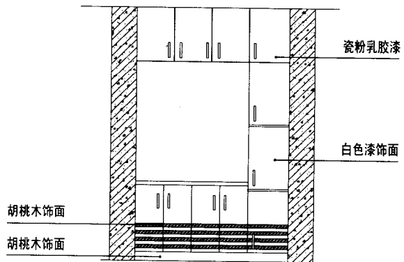
鞋柜立面图
