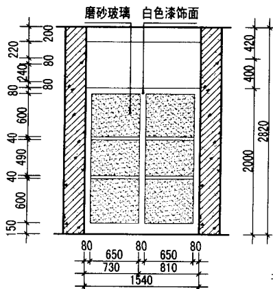
卫生间玻璃横拉门立面图
