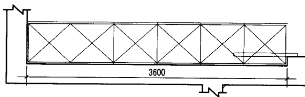
主卧衣柜平面图
