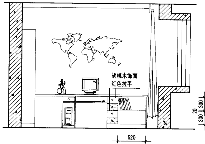
书房电脑桌结构图
