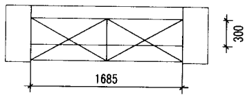
鞋柜平面图
