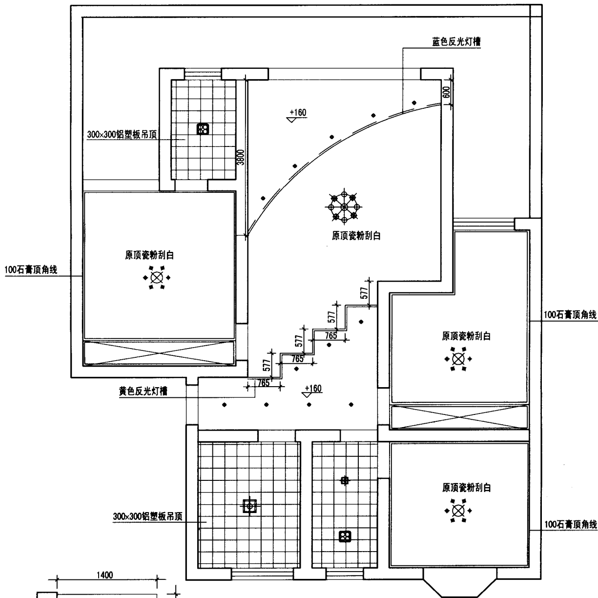
顶面布置图
