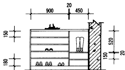
鞋柜结构图
