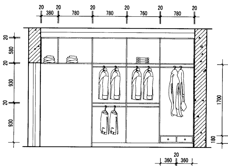
主卧衣柜结构图
