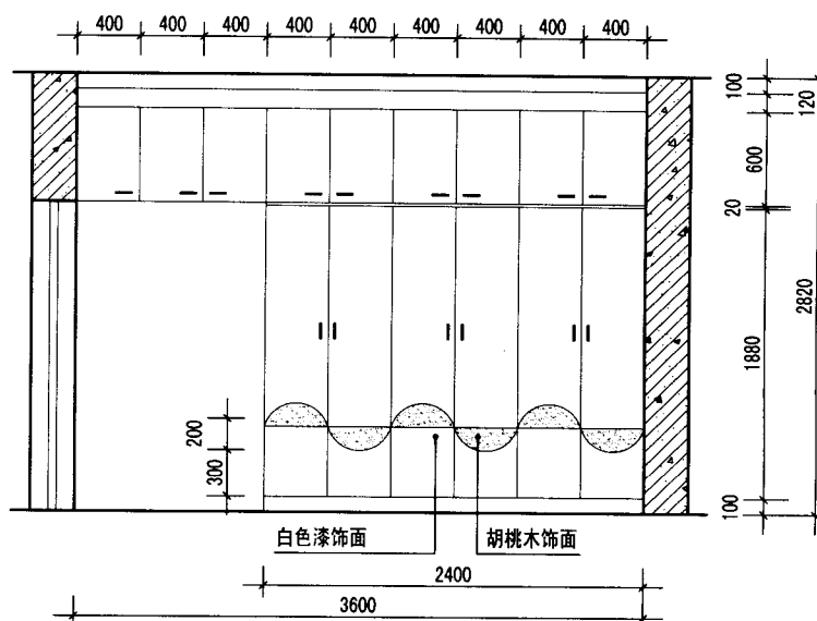
主卧衣柜立面图
