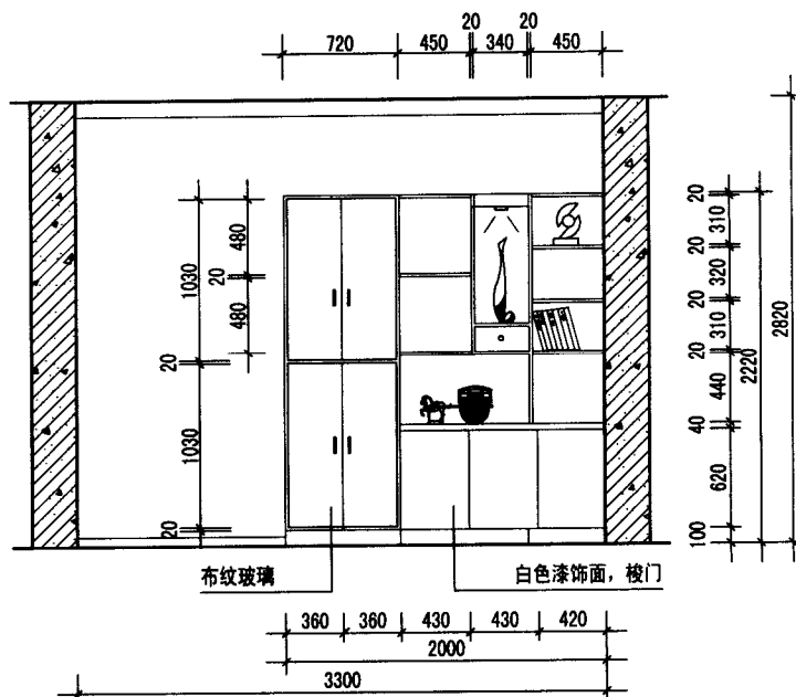
书房书柜立面图
