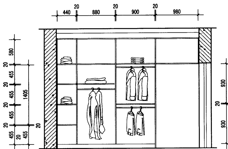
次卧衣柜结构图
