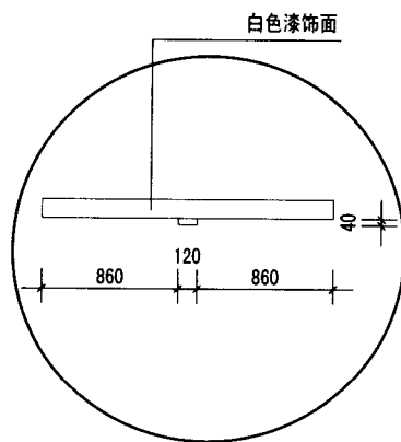
门平面图
