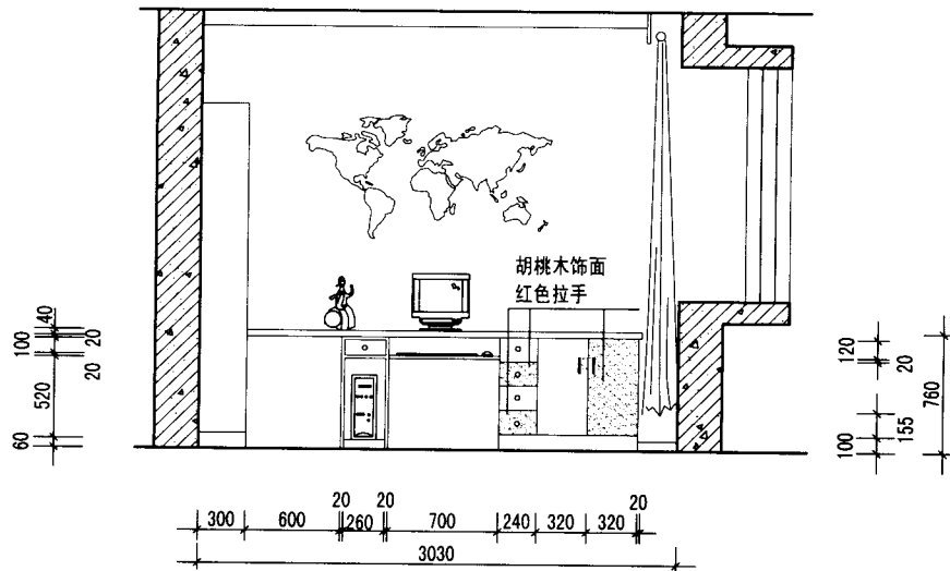
书房电脑桌立面图
