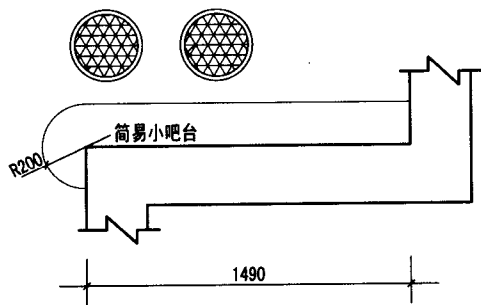
客厅吧台及墙面装饰平面图
