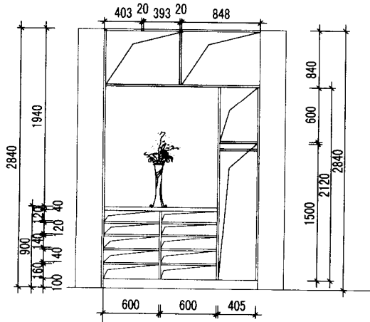
鞋柜结构图
