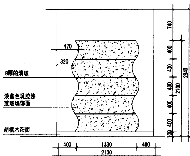
餐厅背景立面图
