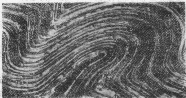
图2 岩层褶皱
