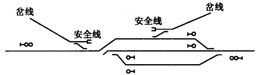
图 1-2 岔线、段管线在站内与正线、到发线接轨
