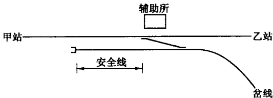
图 1-1 岔线在区间与正线接轨
