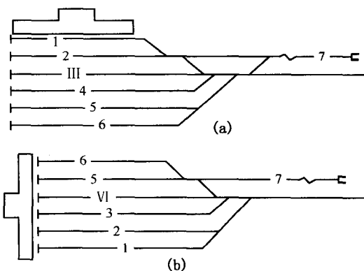
图 1-7 尽头式铁路车站线路编号
