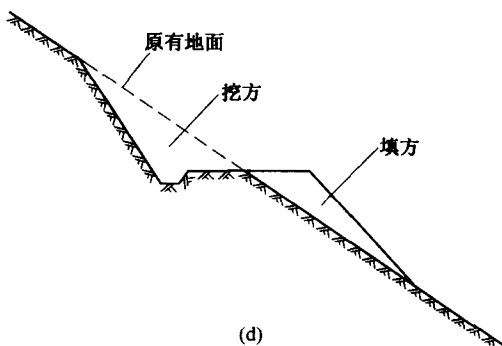
图 1-10 其他路基横断面
