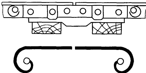
图 1-13 导电接头连接零件
