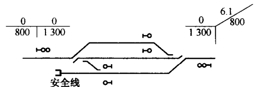
图 1-3 接车线末端设安全线
