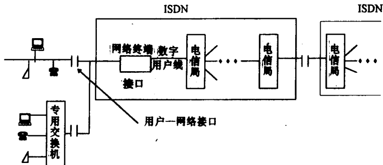
图 1—2 ISDN 的一般结构
