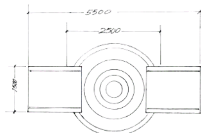
俯视图 1:40
