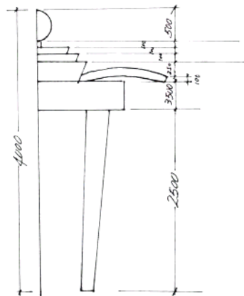
侧视图 1:40
