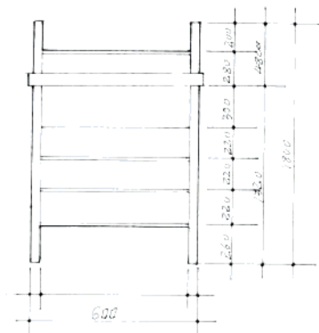
侧立面图
