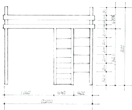
正立面图
