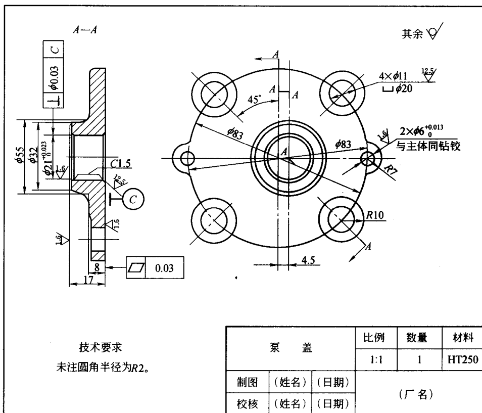
图 1-1 泵盖零件图
