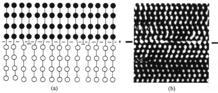
图 5 半共格界面
