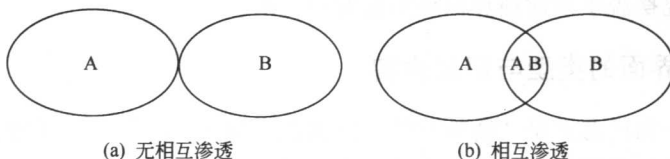
图 2 界面的连接
