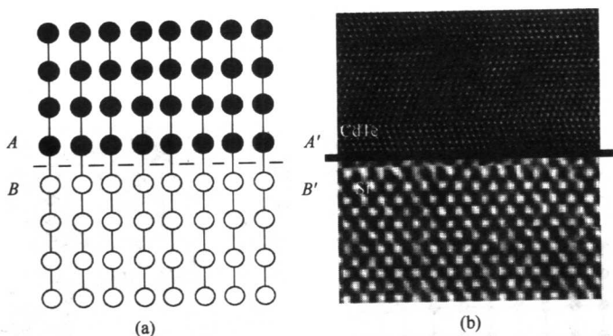
图 4 共格界面
