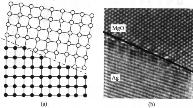
图 6 非共格界面
