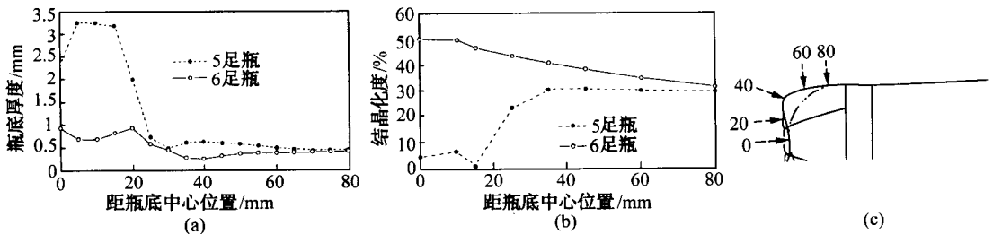
图 1-3 城堡形结构瓶底性能比较图 (a) 瓶底厚度 (b) 瓶底结晶化度 (c) 瓶底距中央部位距离
