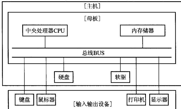
图 1-1-2 计算机的体系结构
