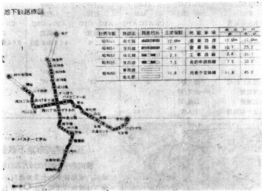
图1—4—1 札幌地下铁道路网规划
