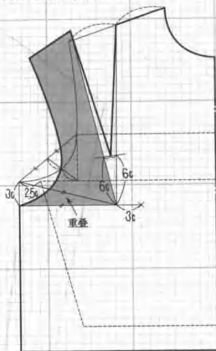
④ 侧省向肩省的移动
