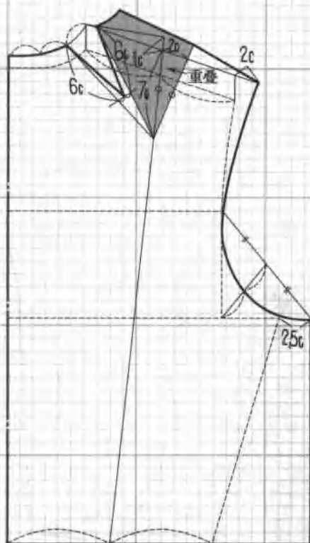
① 后肩省向领省的移动
