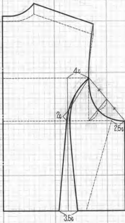
② 后袖窿省与腰省的连接
