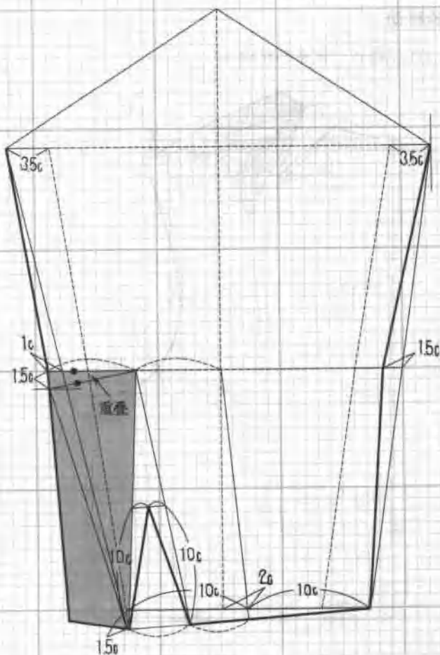
⑥ 袖省向袖口省的移动
