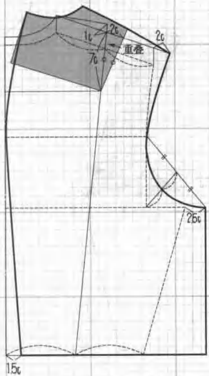
① 后肩省向后中心线省的移动与连接
