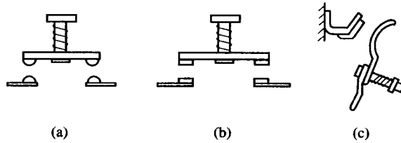
图 1-4 触头的结构形式
