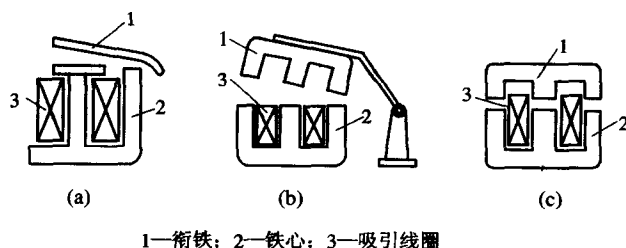
图 1-1 常见的电磁机构
