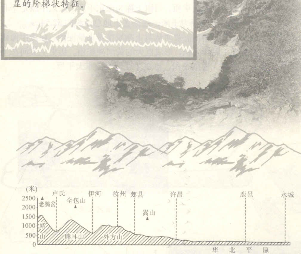
河南地势剖面示意图 (35°N附近)
