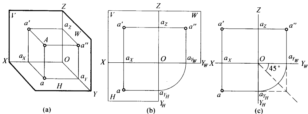
图 2-3 点的三面投影
