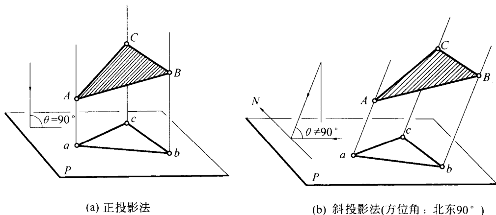
图 1-3 平行投影法
