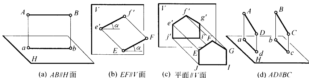
图 1-5 投影的基本性质——不变性
