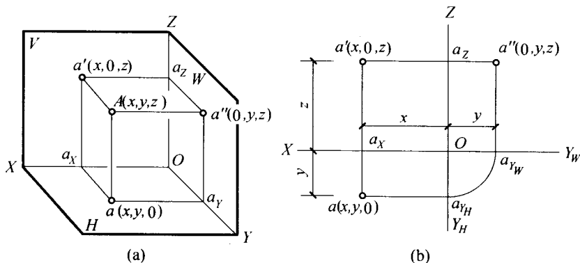
图 2-4 点的投影与坐标
