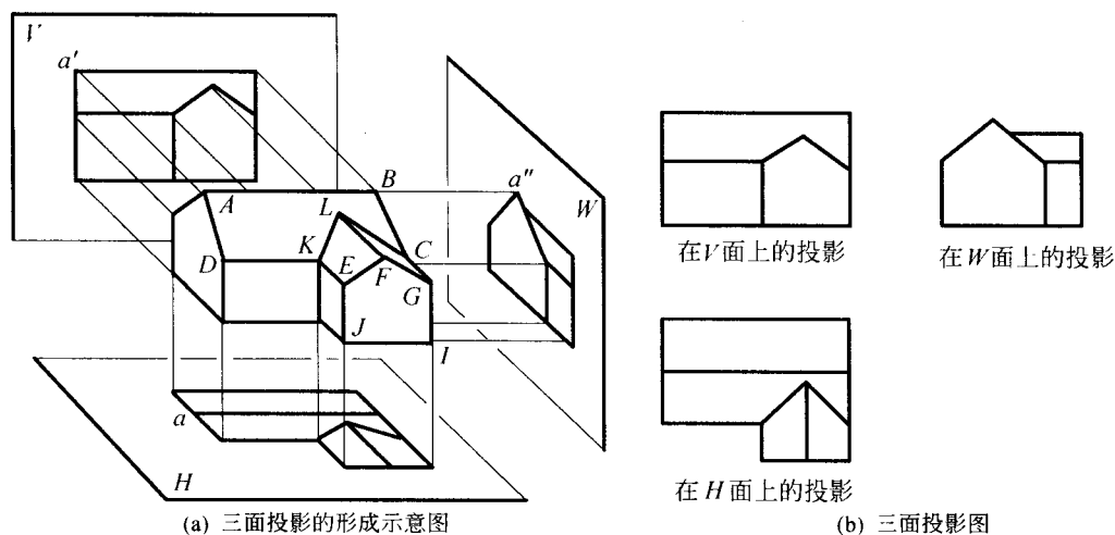
图 1-4 投影的基本性质
