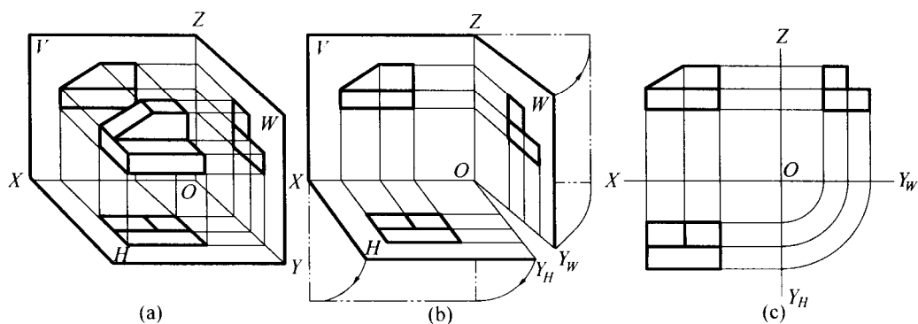
图 1-9 形体的三面投影图
