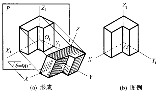
图 1-10 正轴测图
