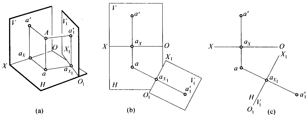
图 2-2 点的辅助投影(一次变换)
