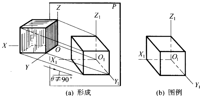
图 1-11 斜轴测图
