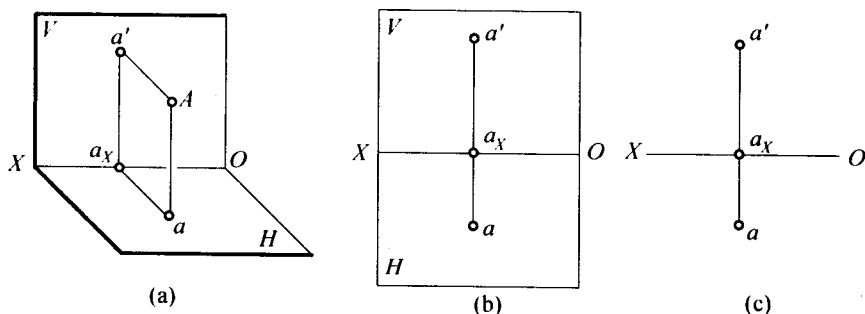
图 2-1 点的两面投影
