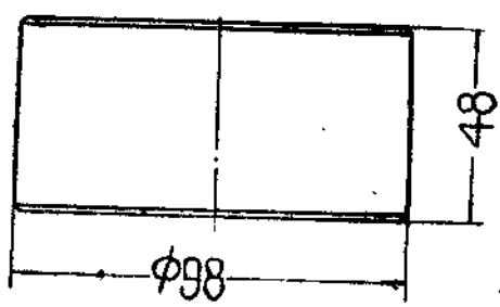
焊接后加工 圆柱 材料15 CП29-11/33-2
