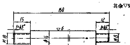
手柄球杆 材料45 CII29-11/22
