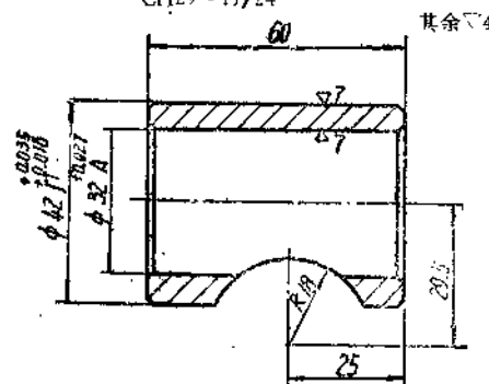
未注尺寸之棱角均为1×45° 套 材料碳钢1 CII29-11/29
