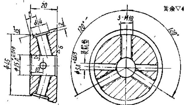
手柄座 材料45 CII29-11/19 表面喷漆 未注尺寸之棱角均为R1
