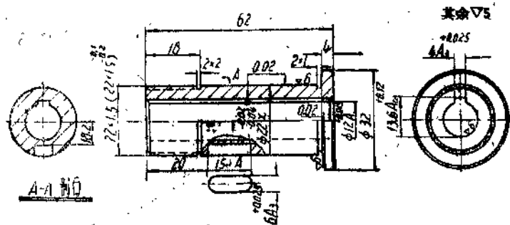
套 材料45 CII29-11/14
