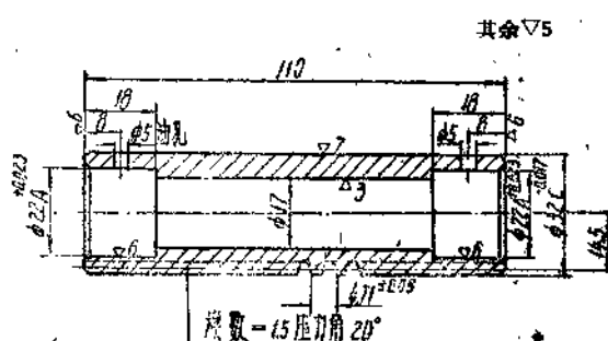
未注尺寸之棱角均为1×45° 套筒 材料45 CII29-11/28
