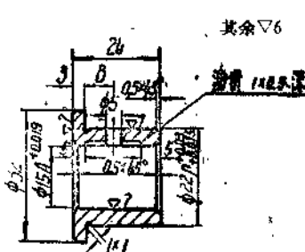
套 材料6-6-3 CII29-11/27
