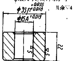
未注尺寸之棱角 均为1×45° 套 材料45 CII29-11/24
