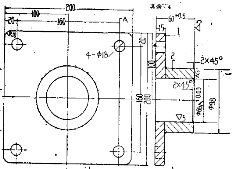
底座焊接圖 CП29-11/33
