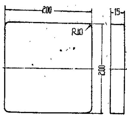
底座 CП29-11/33-1
