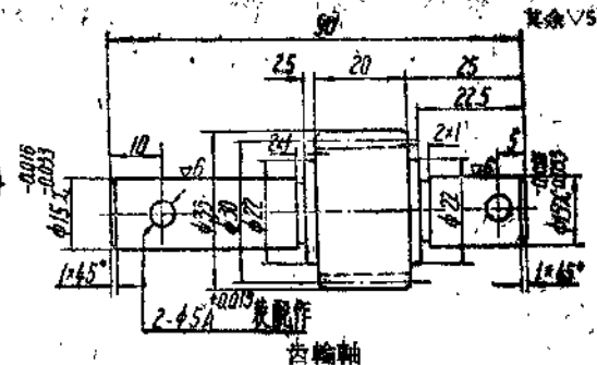
齿轮轴 材料45 CII29-11/20 模数=1.5 压力角=20° 齿数=20
