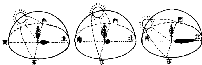
春分、秋分太阳的位置 ↓
