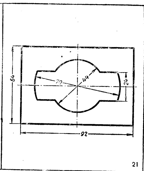
20. 根據已知的尺寸仿製此圖 (圖 21)。
