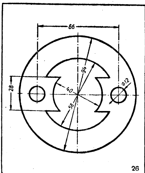
25. 根據已知的尺寸仿製此圖 (圖 26)。
