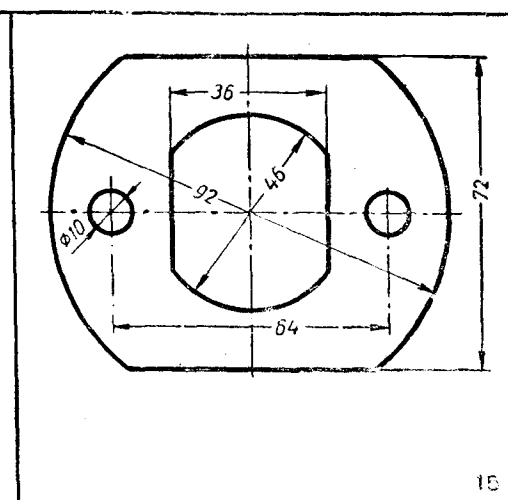
14. 根據已知的尺寸仿製此圖
