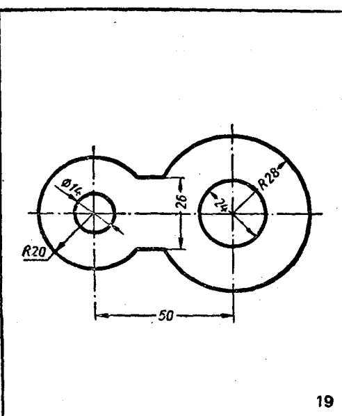
18. 根據已知的尺寸仿製此圖 (圖 19)。
