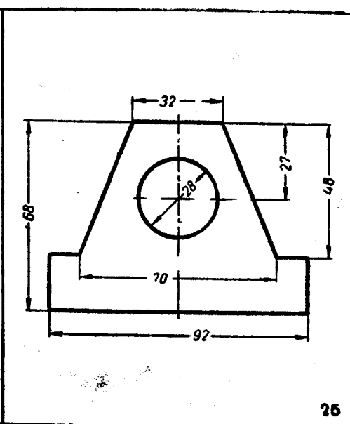
24. 根據已知的尺寸仿製此圖 (圖 25)。
