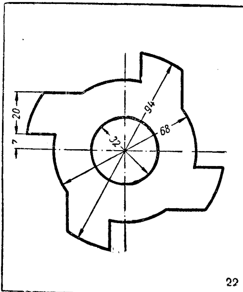
21. 根據已知的尺寸仿製此圖 (圖 22)。
