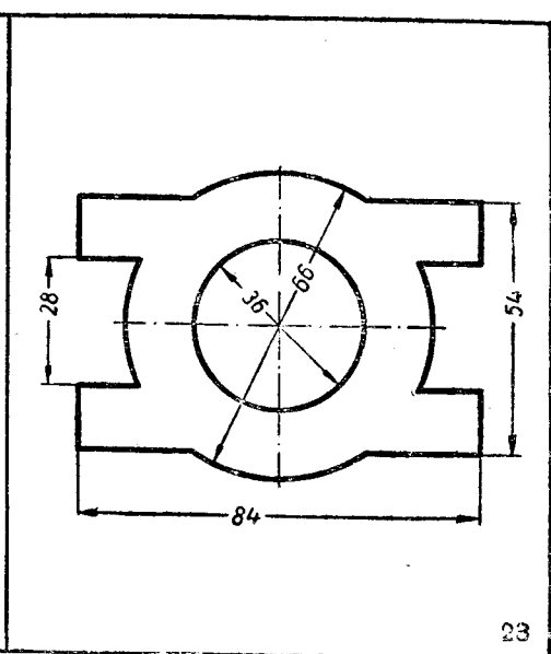
22. 根據已知的尺寸仿製此圖 (圖 23)。
