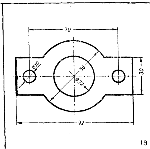
12. 根據已知的尺寸仿製此圖
