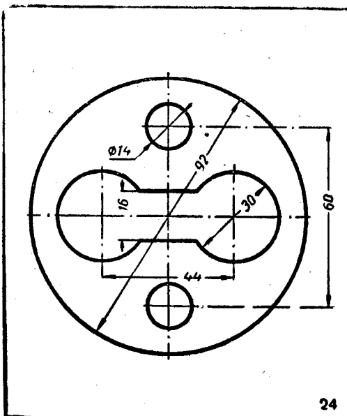
23. 根據已知的尺寸仿製此圖 (圖 24)。
