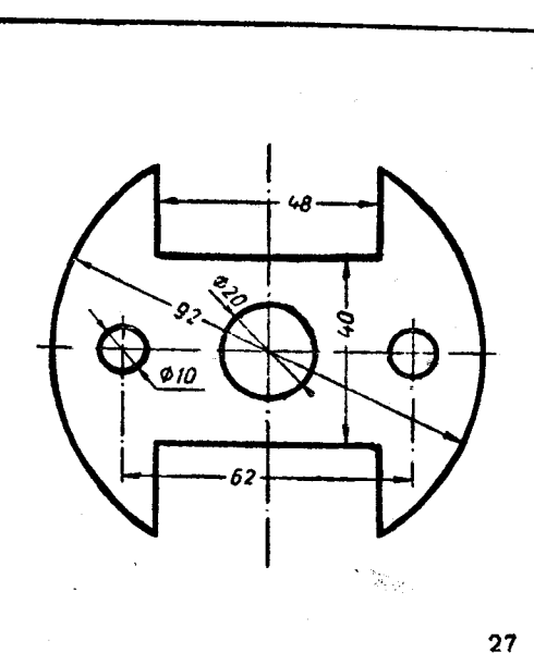
26. 根據已知的尺寸仿製此圖 (圖 27)。
