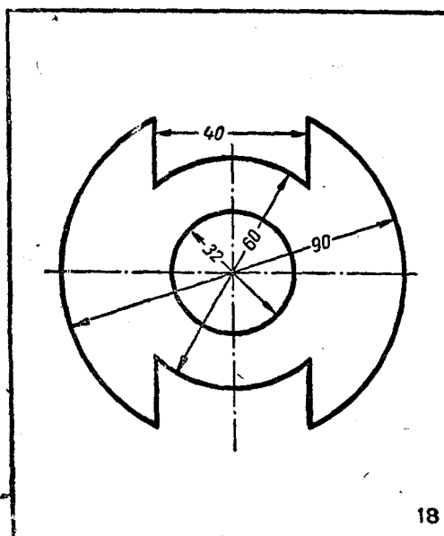
17. 根據已知的尺寸仿製此圖 (圖 18)。
