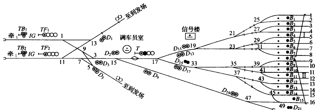
图 1—3 简易和非机械化驼峰示意图
