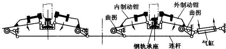
图 1—8 T·JK3 型减速器结构示意图
