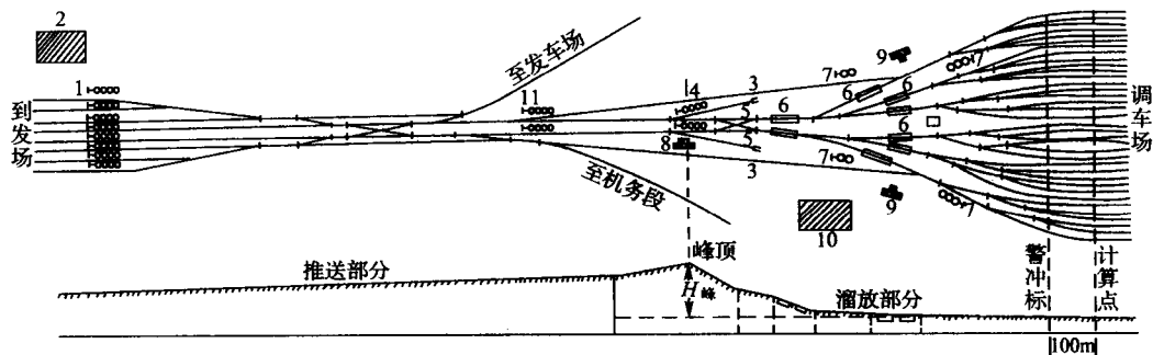
图 1—4 机械化驼峰平、纵断面示意图
