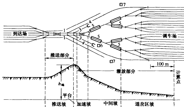
图1—2 驼峰的平、纵断面示意图
