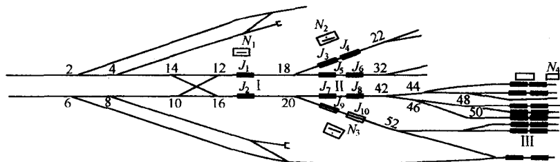
图 1—6 减速器设置地点示意图
