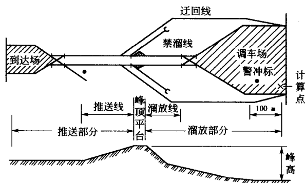
图 1—1 驼峰组成示意图
