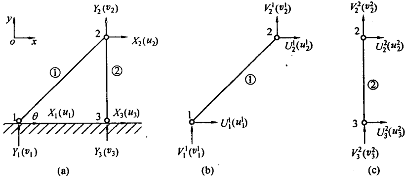
图 1.1 铰接桁架
