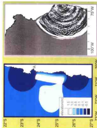
左图：计算机模拟 1995 年 7 月 30 日智利海啸发生时海面的最初状态。A 点为智利安托法加斯塔 (Antofagasta)。右图：计算机模拟同一海啸发生 3 小时后的情形。
