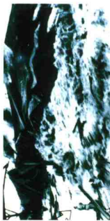
1946 年 4 月 1 日，阿留申群岛地震引发的海啸袭击远在夏威夷群岛的希洛 (Hilo) 港。照片在一艘名为“Higham Vixen”的船上拍摄，显示海啸冲击 1 号码头的情况。相片中左下方的男子最后遇难一劫。(美国国家海洋大气管理局)
