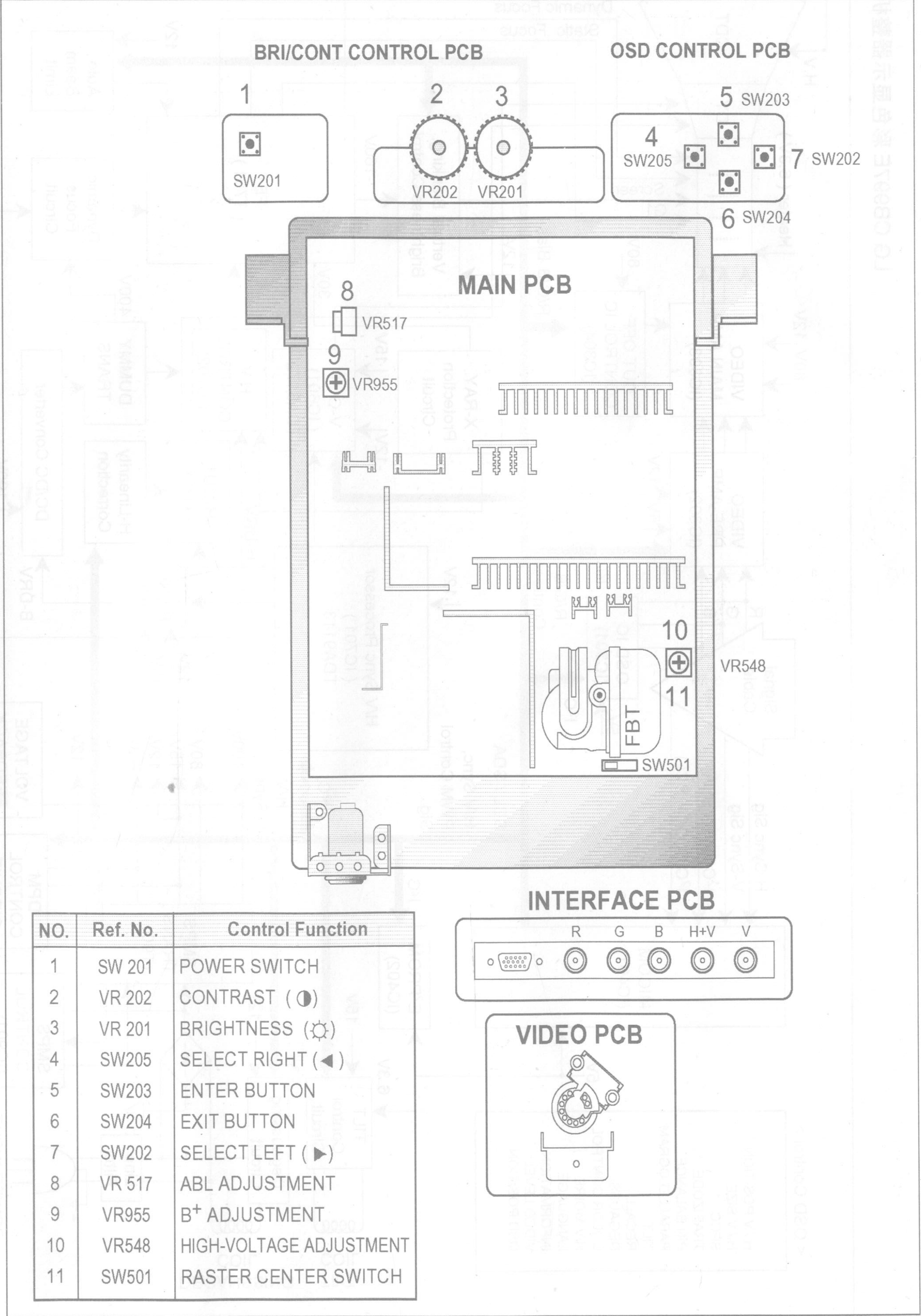
LG CF901 彩色显示器可调元器位置图
