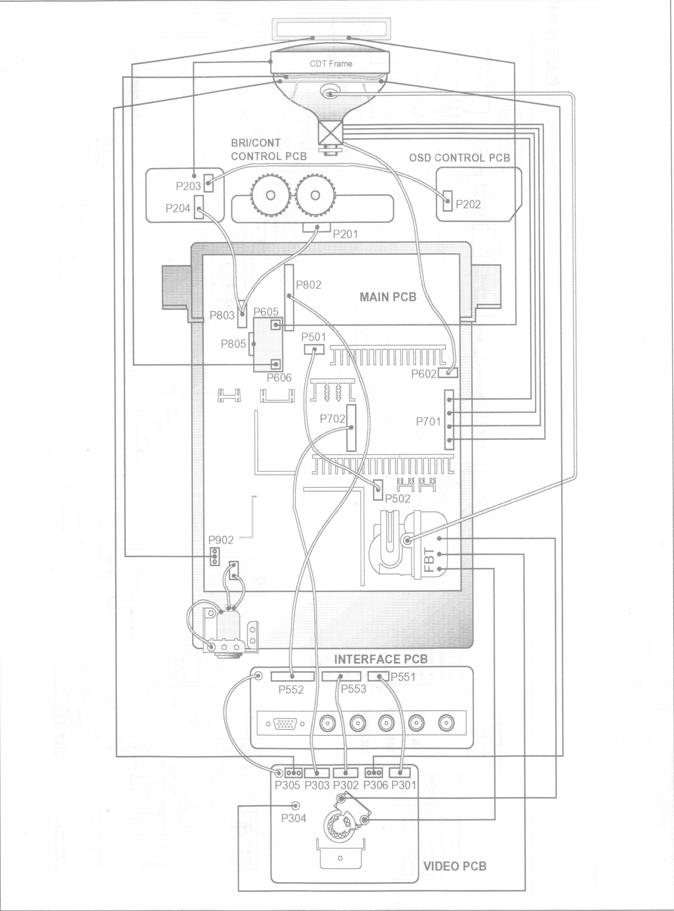
LG CF901 彩色显示器板间接线图
