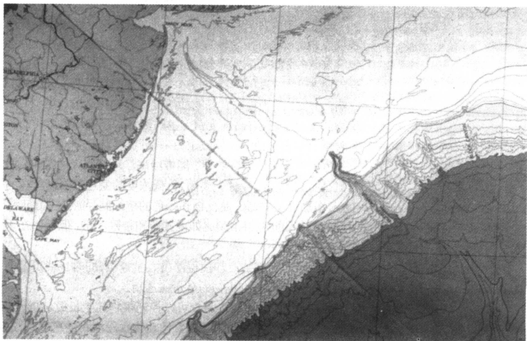
图1.2 这幅纽约湾的地图显示了距美国东北岸宽广的大陆架地区。在大陆架边缘,深海的深度在迅速降低。 (由 Steve Nicklas、美国国家大洋协会、美国国家地理协会和美国国家海洋与大气管理局船只委员会提供图片)
